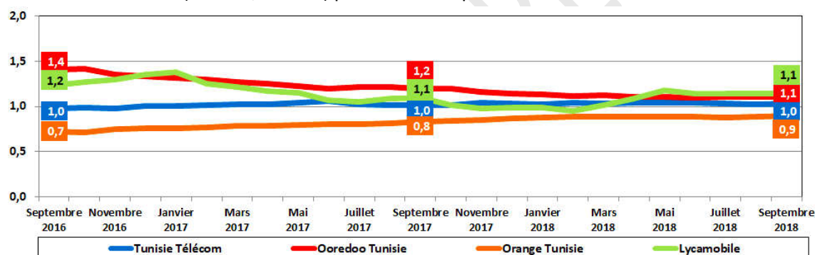
Fig22 : Evolution du rapport Entrant/Sortant par opérateur.
