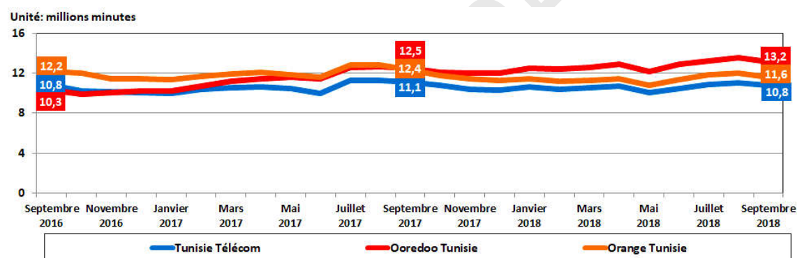
Fig17 : Evolution du trafic journalier moyen par opérateur de la voix mobile off-net.
