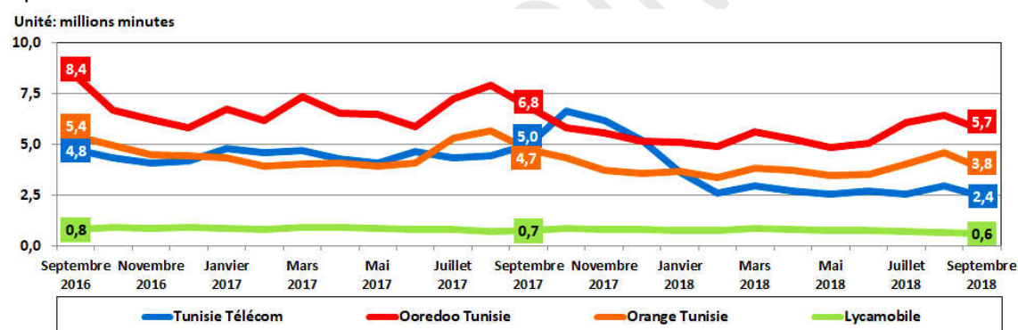
Fig24 : Evolution du trafic voix mobile international sortant par opérateur.
