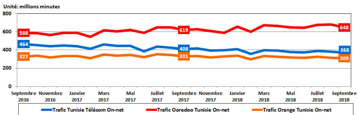
Fig13 : Evolution du trafic voix mobile on-net par opérateur.
